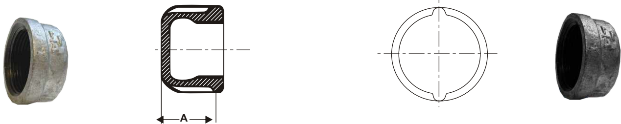
Fig 300 Cap
